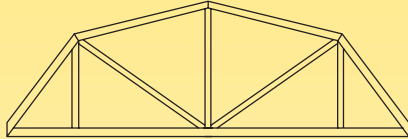
GAMBREL
